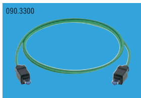
Шнур переключения Real10 Cat.6, S/FTP, 4P, PUR, RJ45/s IP65 type 14-RJ45/s IP65 type 14, 2.5 m Артикул - R501366
