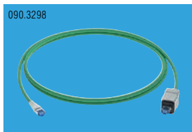
Шнур переключения Real10 Cat.6, S/FTP, 4P, PUR, RJ45/s IP67 type 14-RJ45/s IP20, 2.5 m Артикул - R501366
