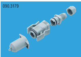
FM45 коннектор Housing IP67, type 06, plastic Артикул - R320691
