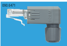
FM45 коннектор IP20, 4P, TIA 568A (AWG26-23), угловой Артикул - R803498
