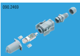
FM45 коннектор IP67, type 06, 4P, TIA 568A (AWG26-23) Артикул - R314686
