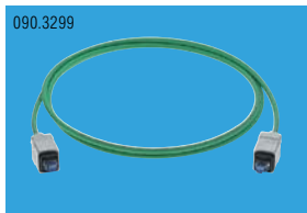
Шнур переключения Real10 Cat.6, S/FTP, 4P, PUR, RJ45/s IP67 type 14-RJ45/s IP67 type 14, 2.5 m Артикул - R501438
