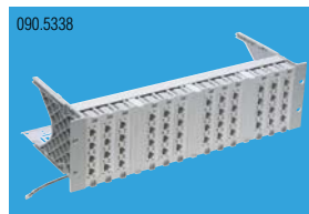
19" 3U Коммутационная панель 48xRJ45/s, Cat.5e, частично заполненная Артикул - R35404
