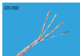
Инсталляционный кабель Cat.5e, SF/UTP, 4P, 200 MHz, PVC, 500 m Артикул - R35052
