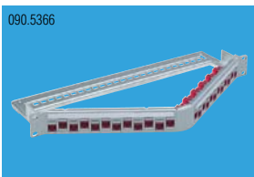
19" 1U Угловая коммутационная панель 24xRJ45/u, Cat.6A ISO, серая Артикул - R509885
